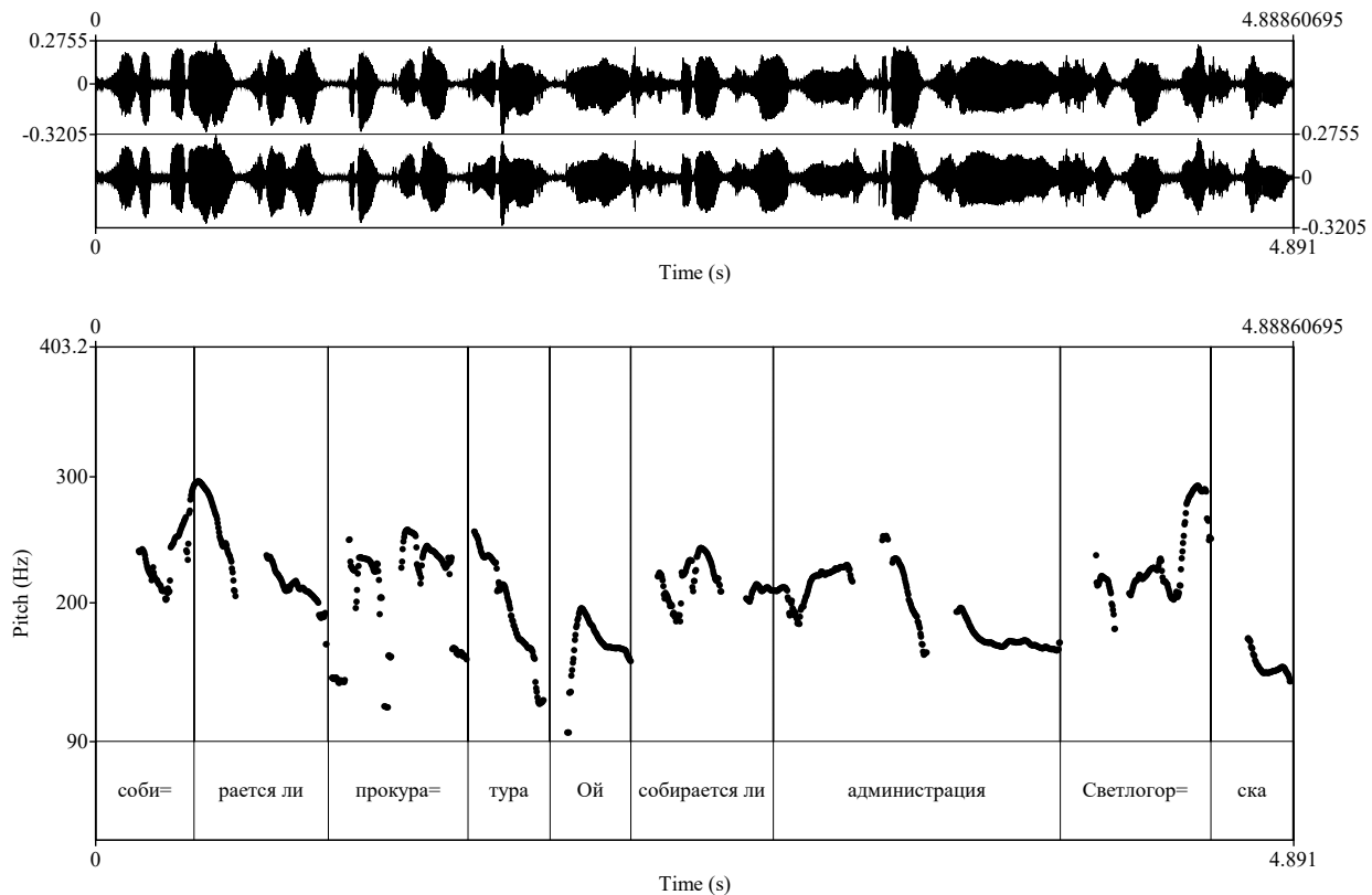
Рисунок 4. Осциллограмма и интонограмма примера (7)
