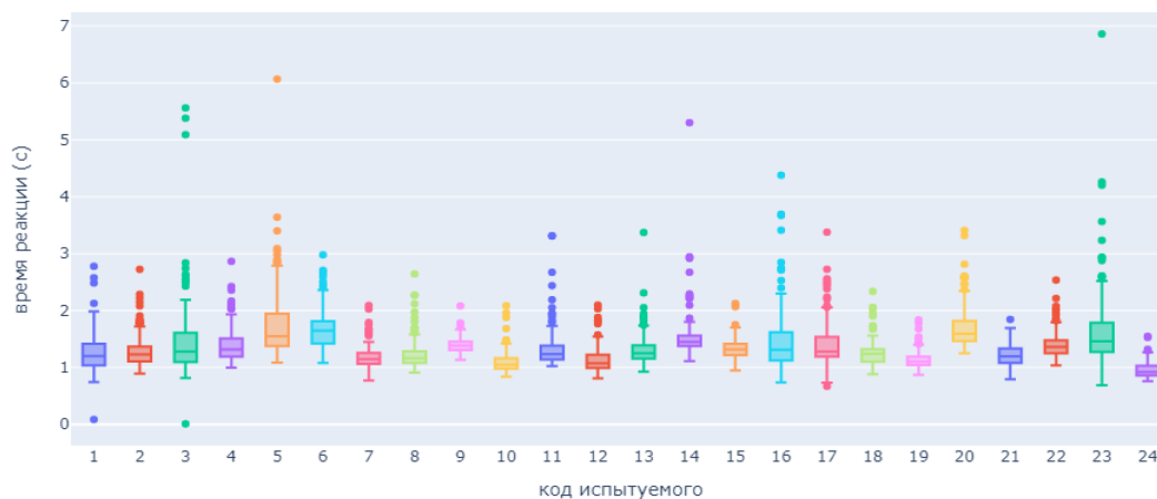
Рисунок 6: распределение времени реакции на псевдослова по испытуемым
