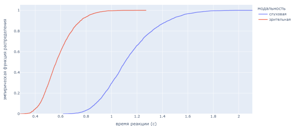
Рисунок 11: графики эмпирических функций распределения времени реакции на слова в ЗМ (красный) и СМ (синий)
