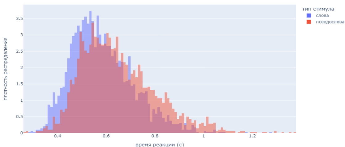
Рисунок 3: гистограммы плотности распределения времени реакции на слова (синий) и псевдослова (красный)
