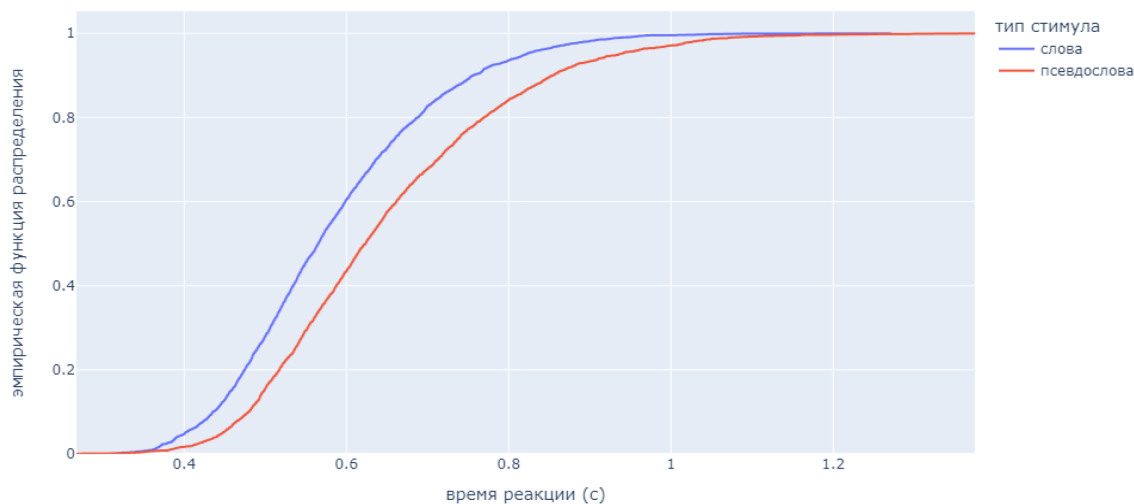
Рисунок 4: графики эмпирических функций распределения времени реакции на слова (синий) и псевдослова (красный)
