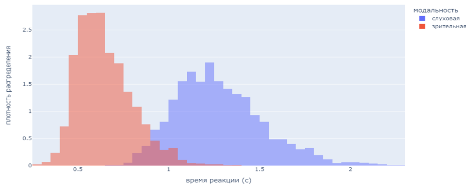
Рисунок 10: гистограммы плотности распределения времени реакции на псевдослова в ЗМ (красный) и СМ (синий)
