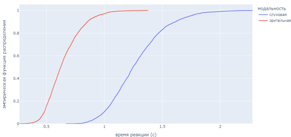
Рисунок 12: графики эмпирических функций распределения времени реакции на псевдослова в ЗМ (красный) и СМ (синий)
