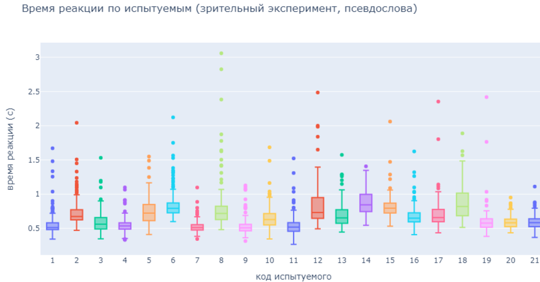
Рисунок 2: распределение времени реакции на псевдослова по испытуемым
