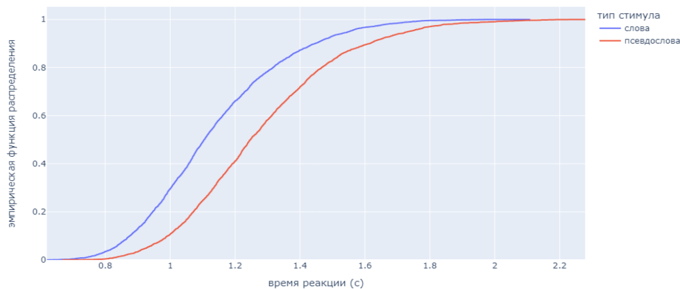
Рисунок 8: графики эмпирических функций распределения времени реакции на слова (синий) и псевдослова (красный)
