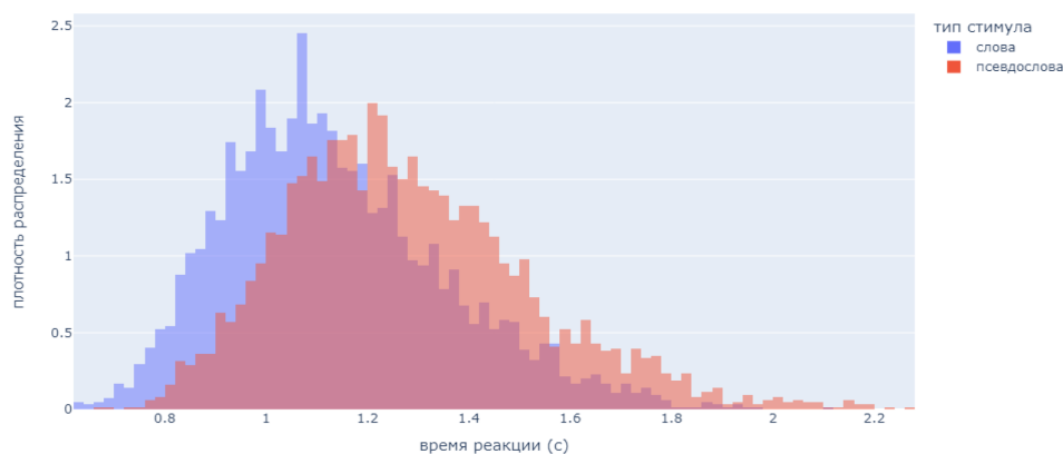
Рисунок 7: гистограммы плотности распределения времени реакции на слова (синий) и псевдослова (красный)
