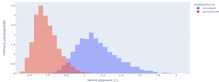
Рисунок 9: гистограммы плотности распределения времени реакции на слова в ЗМ (красный) и СМ (синий)
