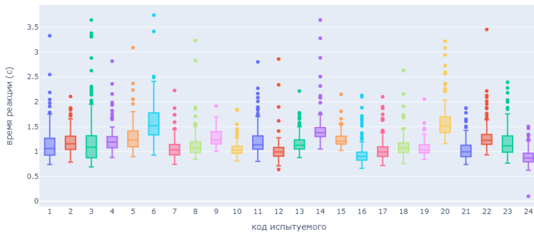
Рисунок 5: распределение времени реакции на слова по испытуемым
