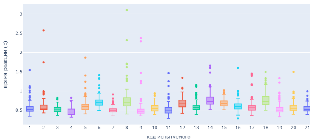
Рисунок 1: распределение времени реакции на слова по испытуемым
